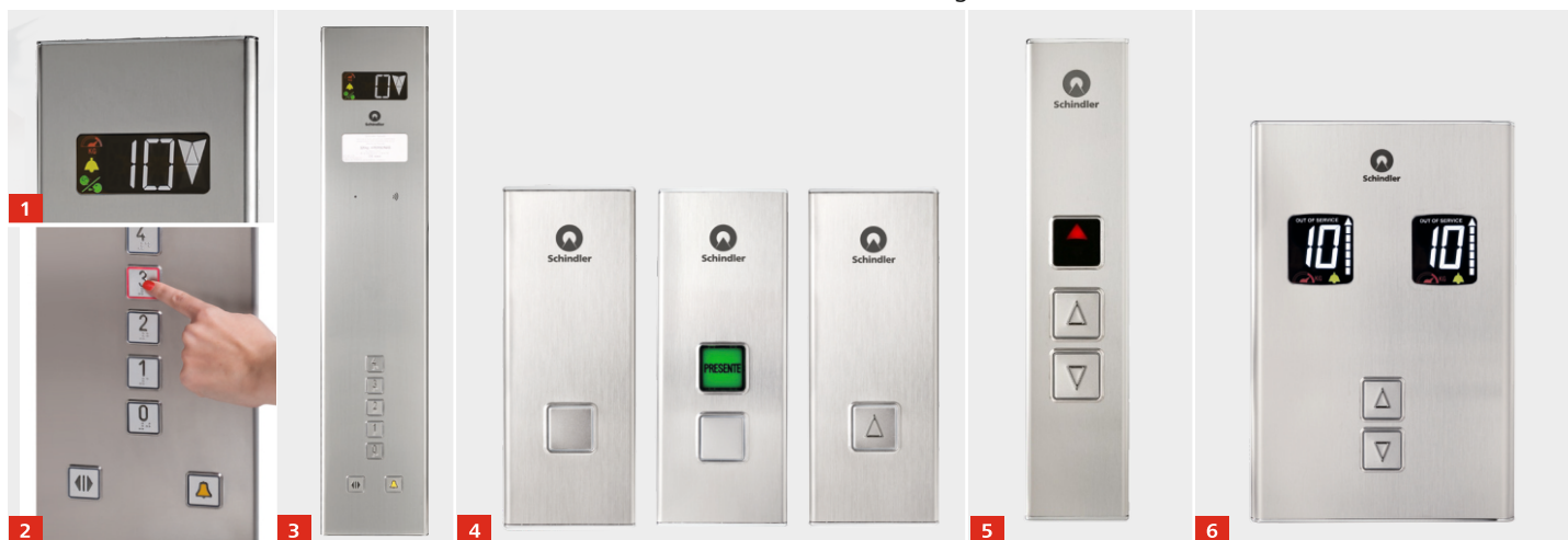
1: Indicador LED na cabina | 2: Detalhe botoneira de cabina | 3: Botoneira de cabina | 4: Botoneiras de patamar | 5: Botoneiras de patamar com indicador de direção | 6: Botoneiras de patamar para dúplex com indicador
